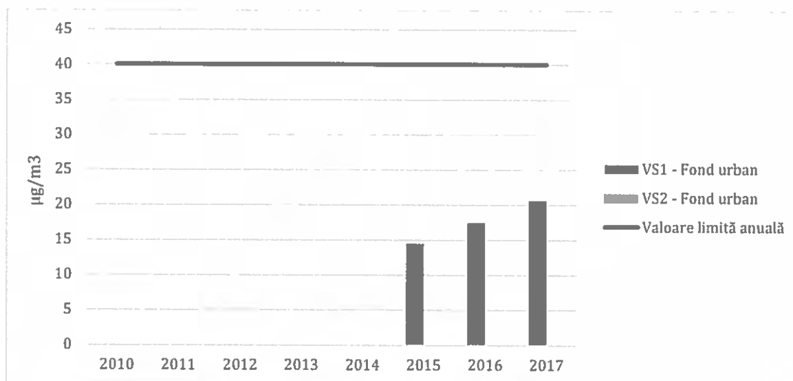
Figura nr. 3-5 - Concentrații medii anuale pentru dioxid de azot ( \text{NO}_2 ), înregistrate la stațiile de monitorizare din județul Vaslui, în raport cu valoarea limită anuală pentru protecția sănătății umane
