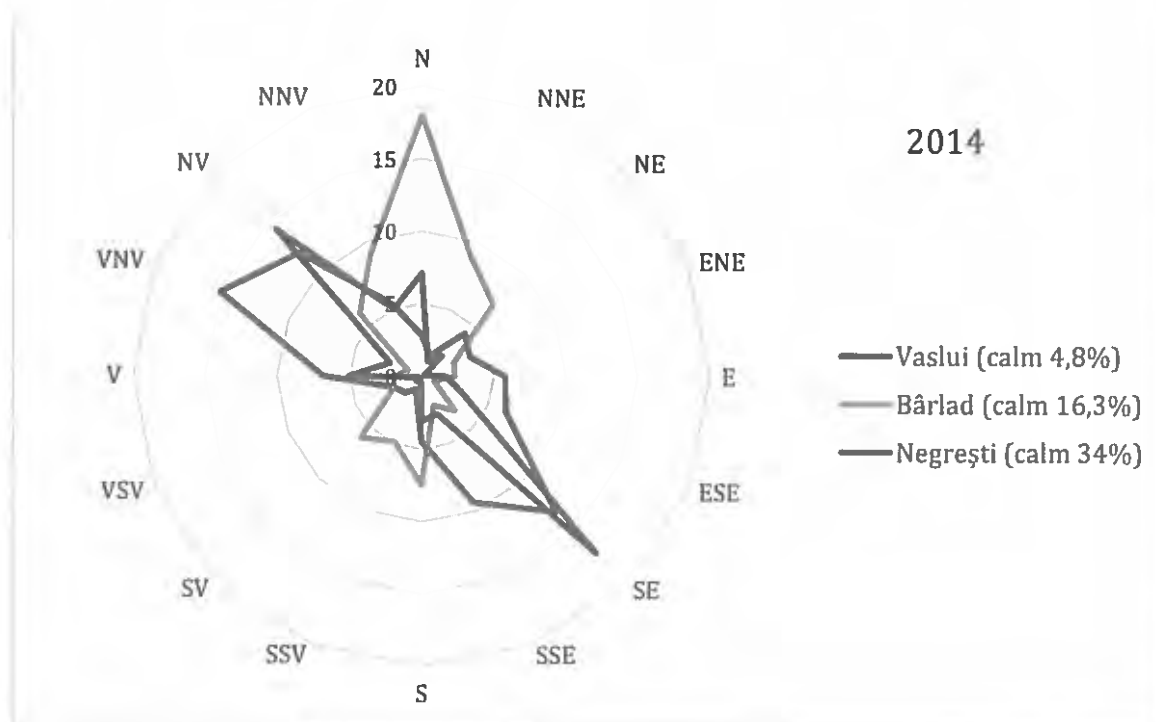
Figura nr. 3-26 - Roza vânturilor medii pentru județul Vaslui, anul 2014
