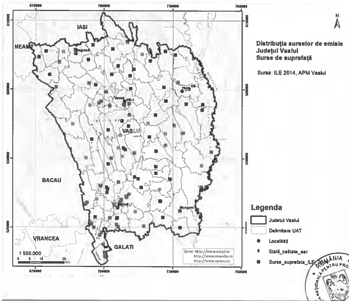
Figura nr. 3-19 - Surse emisii de suprafață în județul Vaslui (ILE 2014)
