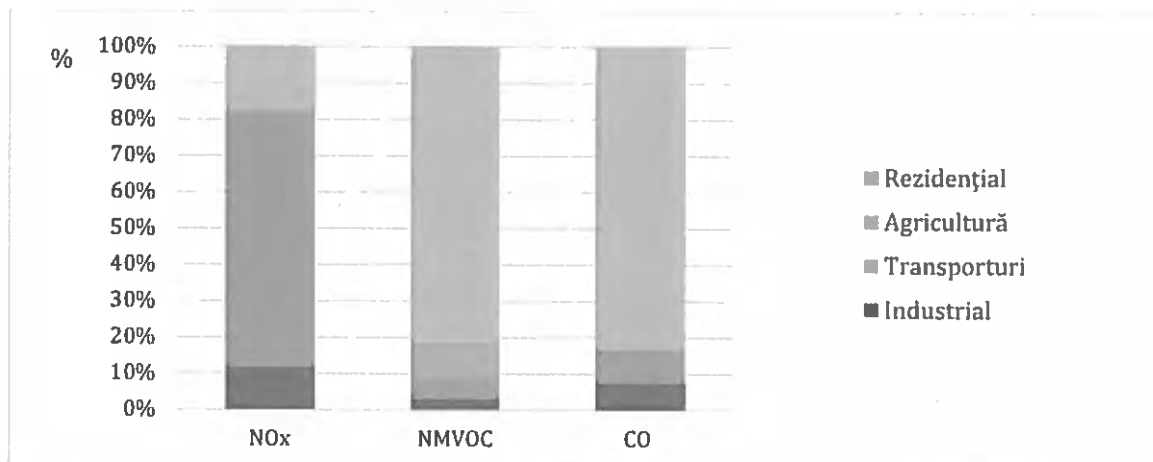
Figura nr. 3-30 - Contribuția sectoarelor de activitate la emisiile de poluanți precursori ai ozonului, la nivelul județului Vaslui, în anul 2014
