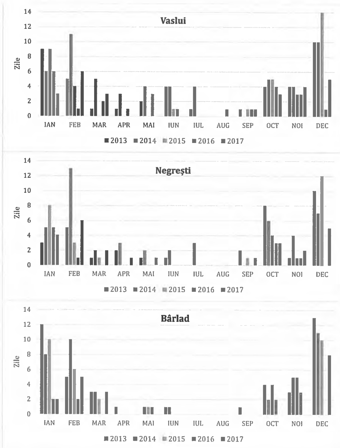
Figura nr. 3-23 - Numărul de zile din lună în care a avut loc fenomene de ceață, în perioada 2013-2017, la stațiile meteorologice din județul Vaslui
