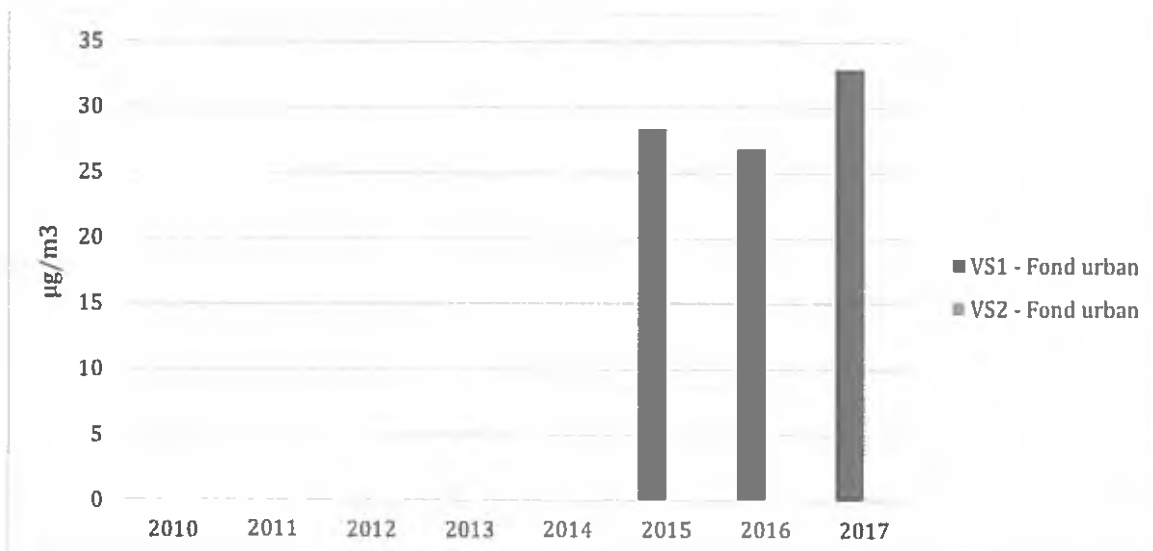
Figura nr. 3-6 - Concentrații medii anuale pentru oxizi de azot ( \text{NO}_x ), înregistrate la stațiile de monitorizare din județul Vaslui
