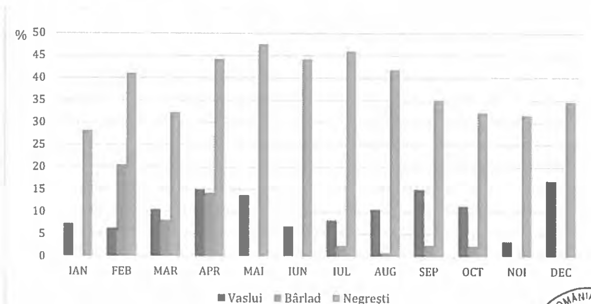
Figura nr. 3-29 – Calmul atmosferic înregistrat la stațiile meteorologice din zona studiată, în anul 2014
