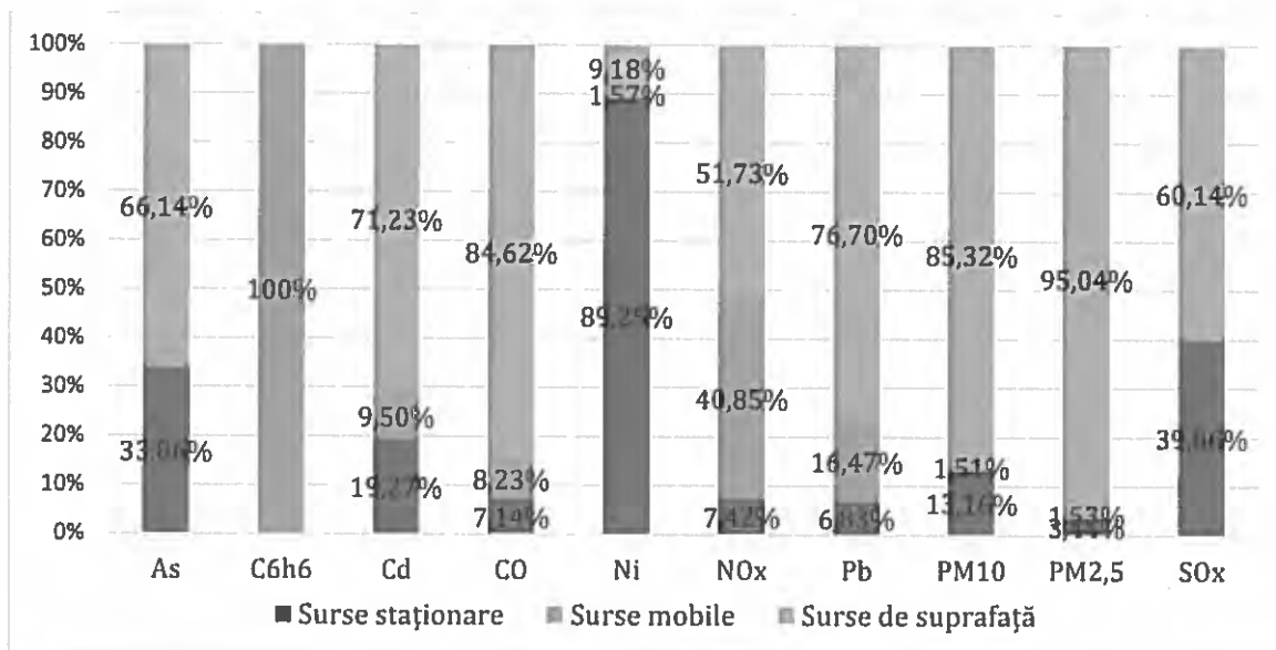
Figura nr. 3-13 - Contribuția diferitelor categorii de surse la emisiile de poluanți în atmosferă, în județul Vaslui, în anul de referință 2014
