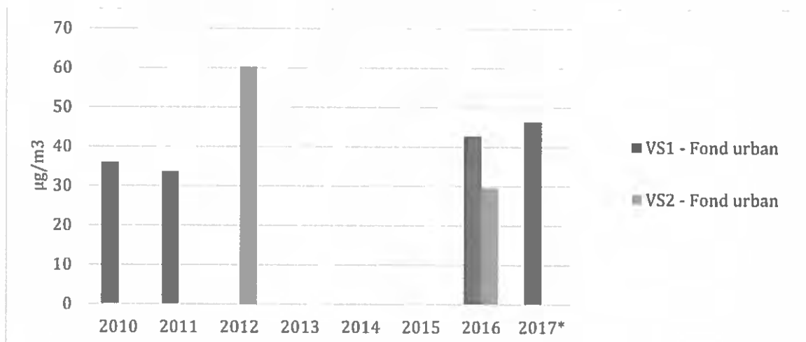
Figura nr. 3-32 - Evoluția concentrațiilor medii anuale ale ozonului (O 3 ) înregistrate la stațiile de monitorizare din județul Vaslui
