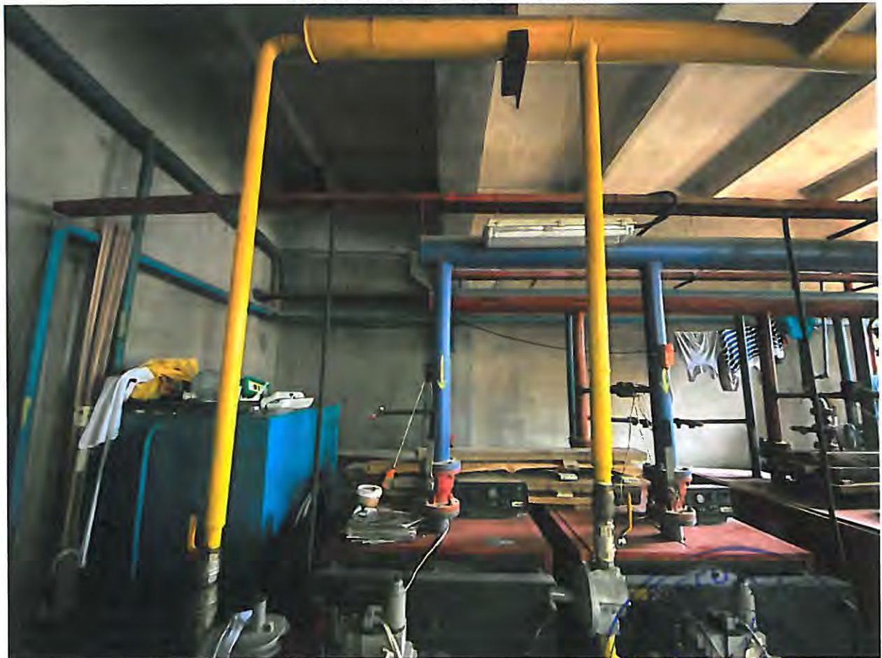
FOTO CENTRALĂ TERMICĂ
