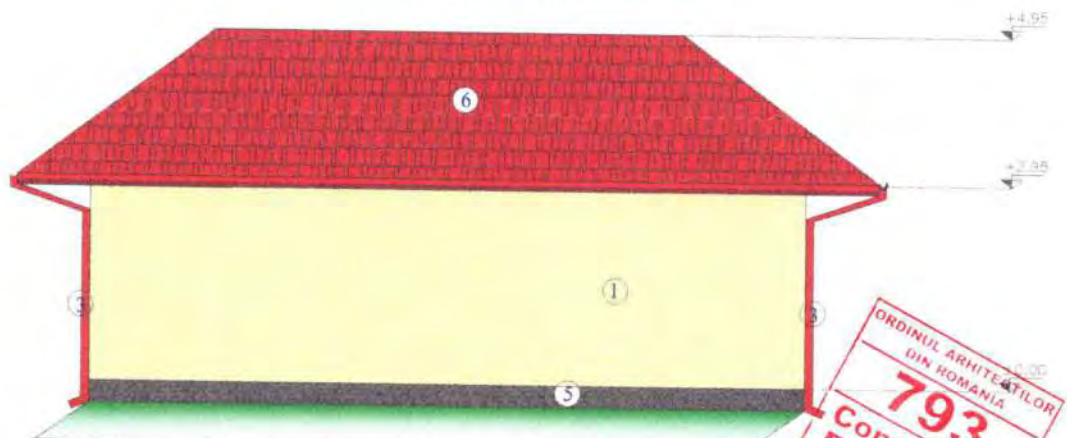
FATADA POSTERIOARA
